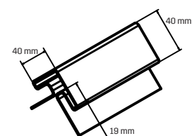
NAROŻNIK ZEWNĘTRZNY
